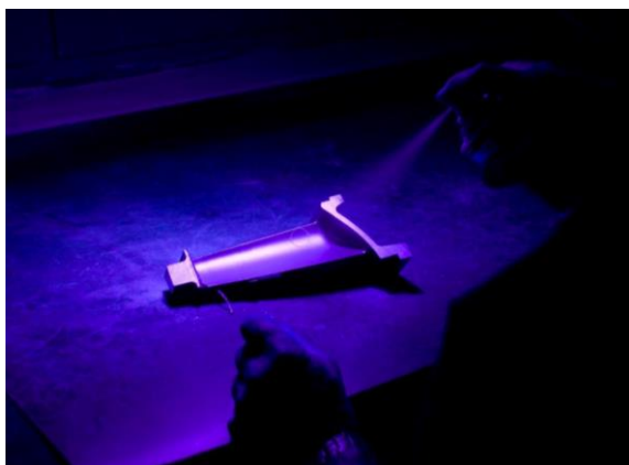
Неразрушающий контроль
